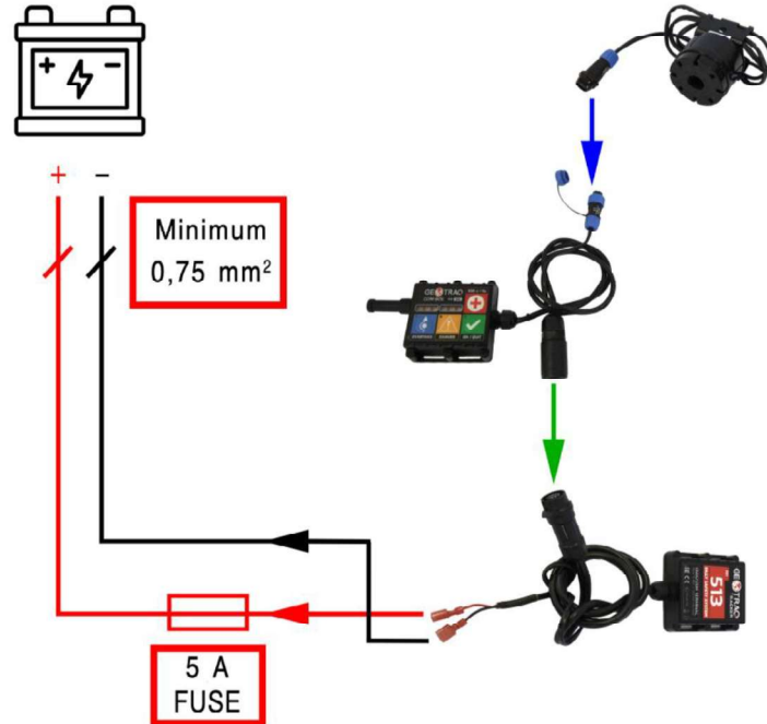
Sistem bağlantı şeması
